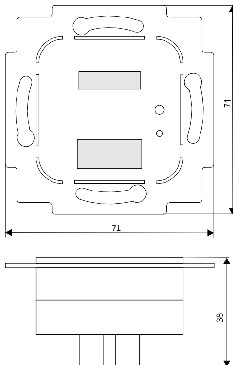
RS485-Schnittstelle RS485-Interface
